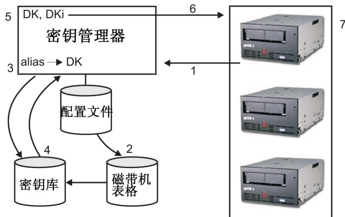
图 2-1. LTO 4 或 LTO 5 磁带机请求加密写操作
